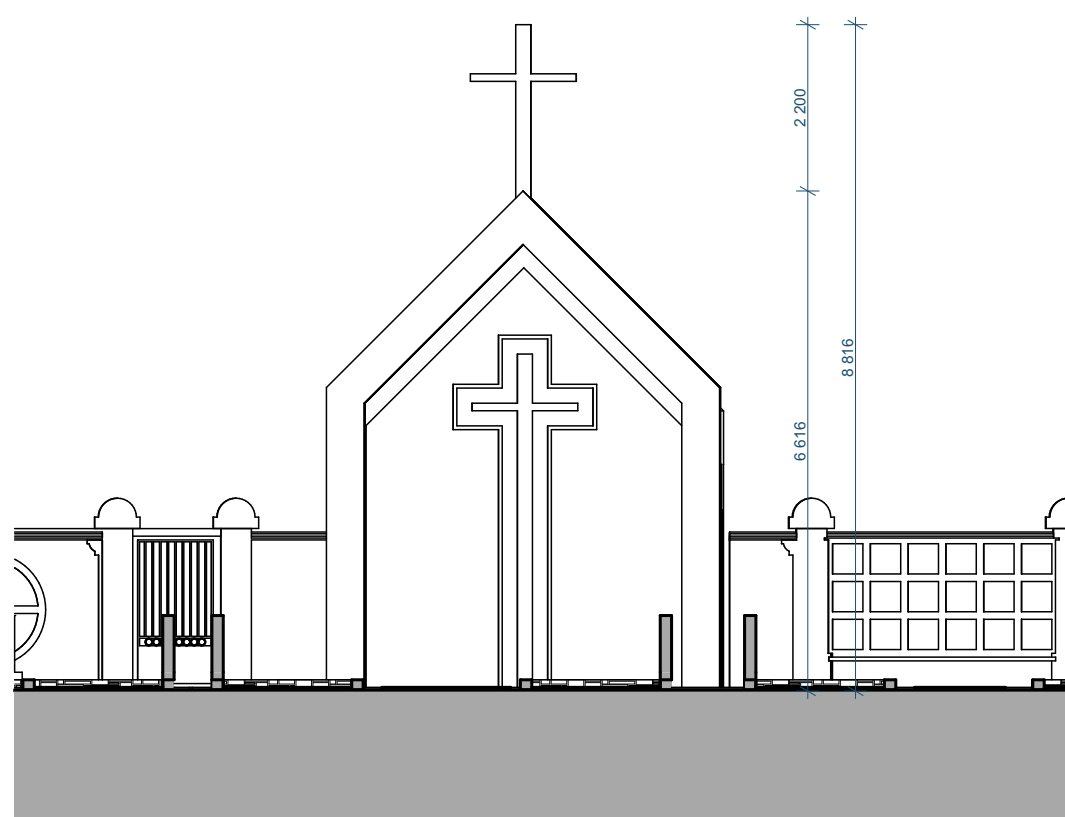
KAPLE POHLED ČELNÍ - NAVRHOVANÝ STAV.
