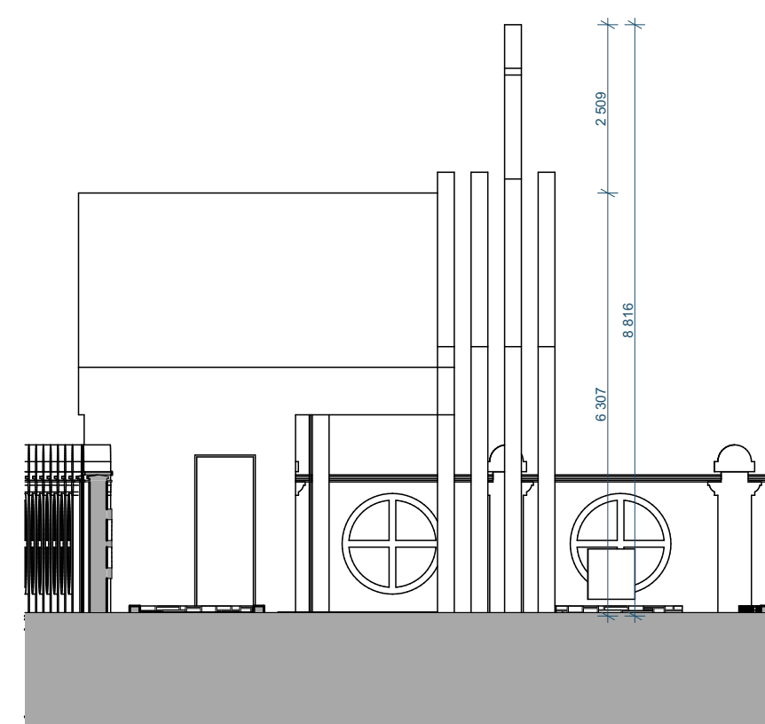
KAPLE POHLED BOČNÍ LEVÝ - NAVRHOVANÝ STAV.
