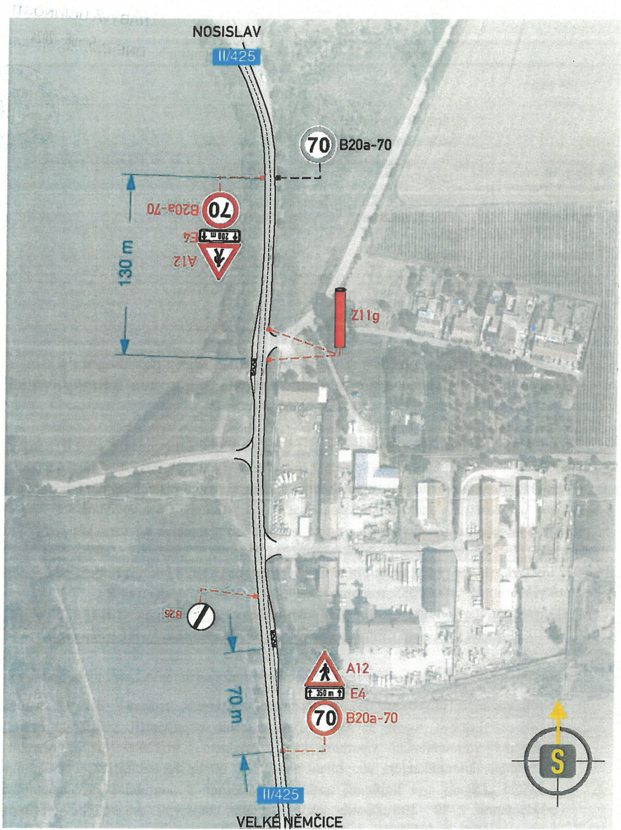
Obrázek 1: Situace dopravního značení
